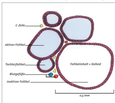
Schematischer Querschnitt durch Schilddrüsenzellen. Die Reichweite der Strahlung entspricht etwa 0,5 mm, also ungefähr einem Zelldurchmesser.
